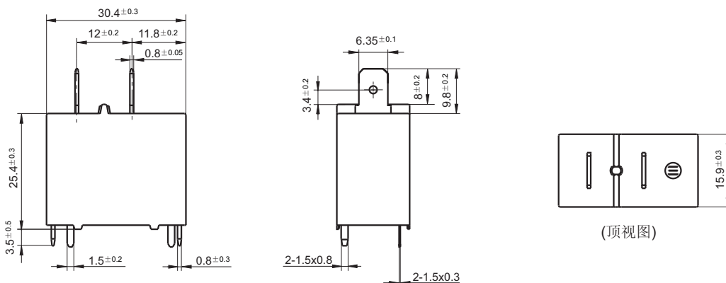
外形图
